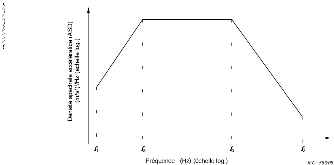
Figure A.1 – Points aux fréquences de transfert pour le spectre – Transport
