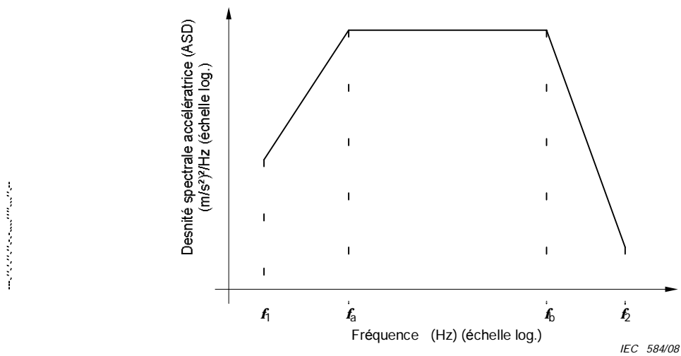
Figure A.2 – Points aux fréquences de transfert pour le spectre – Installations fixes
